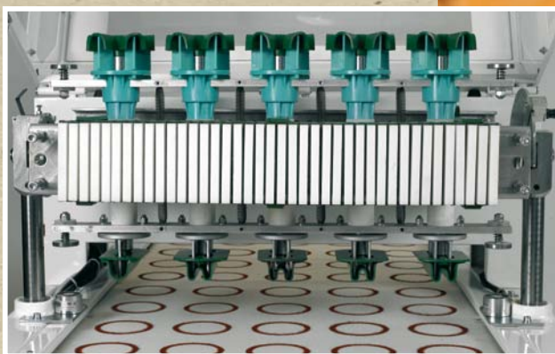
Barra ventaglio Fan-shaped bar Barre "ventaglio"
